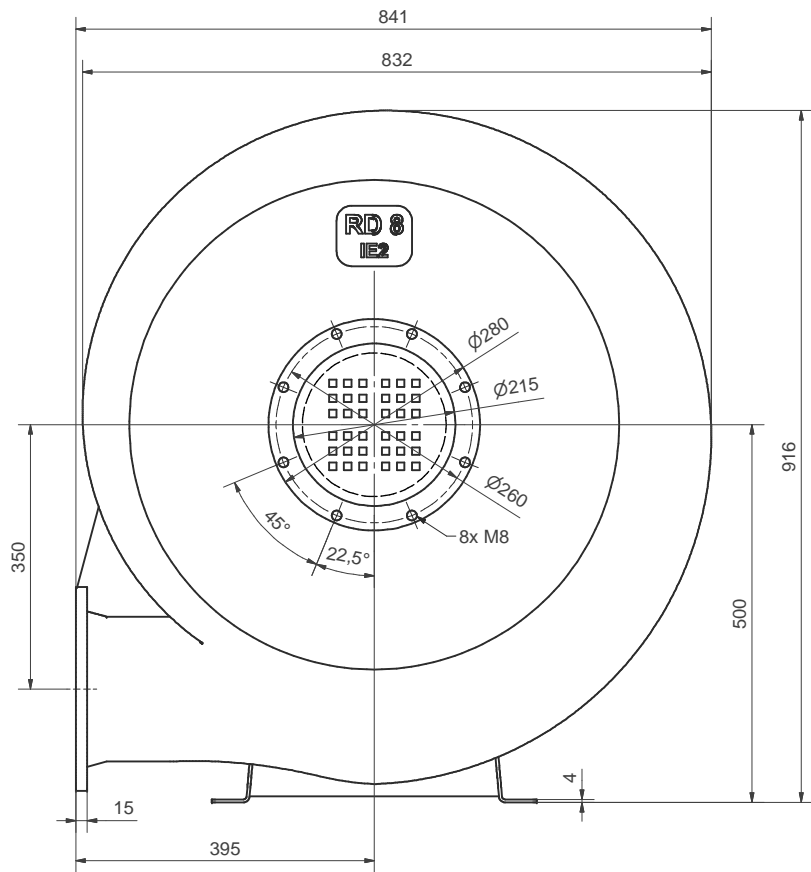
↑ Ansicht A
