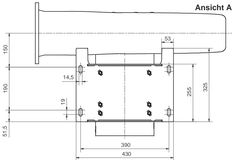
↑ Ansicht A
