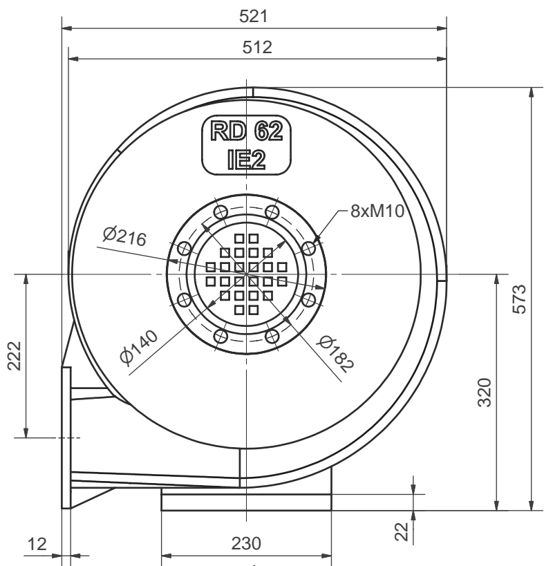
Ansicht A
